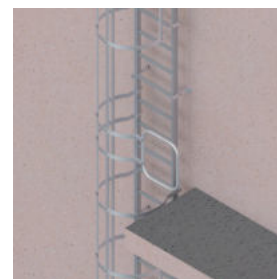
Selbstschließende Türe zu Steigleiter für Seitenausstieg
