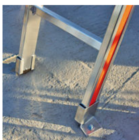
Paar Bodenwinkel für Sprossenleitern für Profil 70
